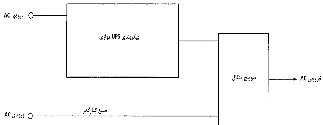
شکل ۴-۲۳: UPS موازی با کنارگذر و سوئیچ انتقال
