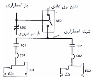
شکل ۲-۳: دو دستگاه موتور - ژنراتور با اتصال موازی
