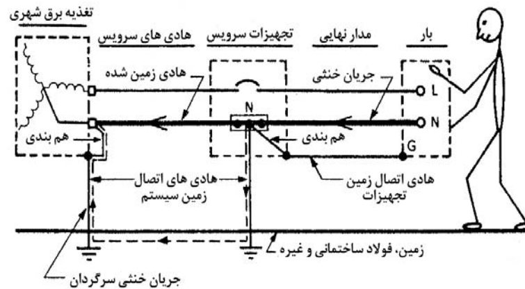
شکل ۴-۶: جریان خنثی سرگردان به علت زمین شده چندانکه هادی سرویس زمین شده
