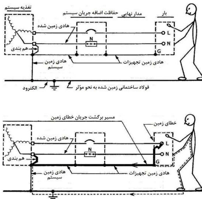
شکل ۶-۱: اتصال زمین سیستم و تجهیزات - نوع یکپارچه - برای سیستم با منبع تغذیه سرویس
