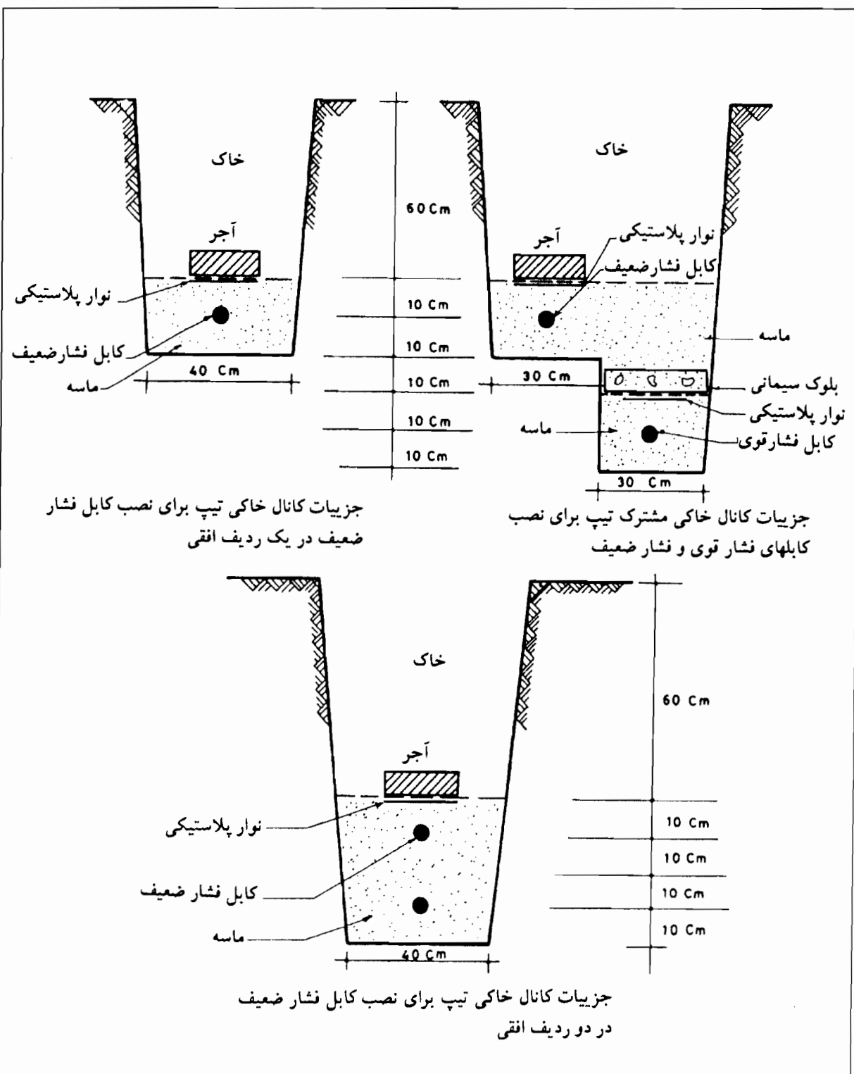
جدول ابعاد کانالهای خاکی بر حسب تعداد و نوع استقرار کابل های فشار ضعیف
