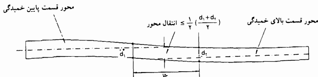
شکل ۱۳-۳ خمیدگی کوتاه تیر، حالت اول.
