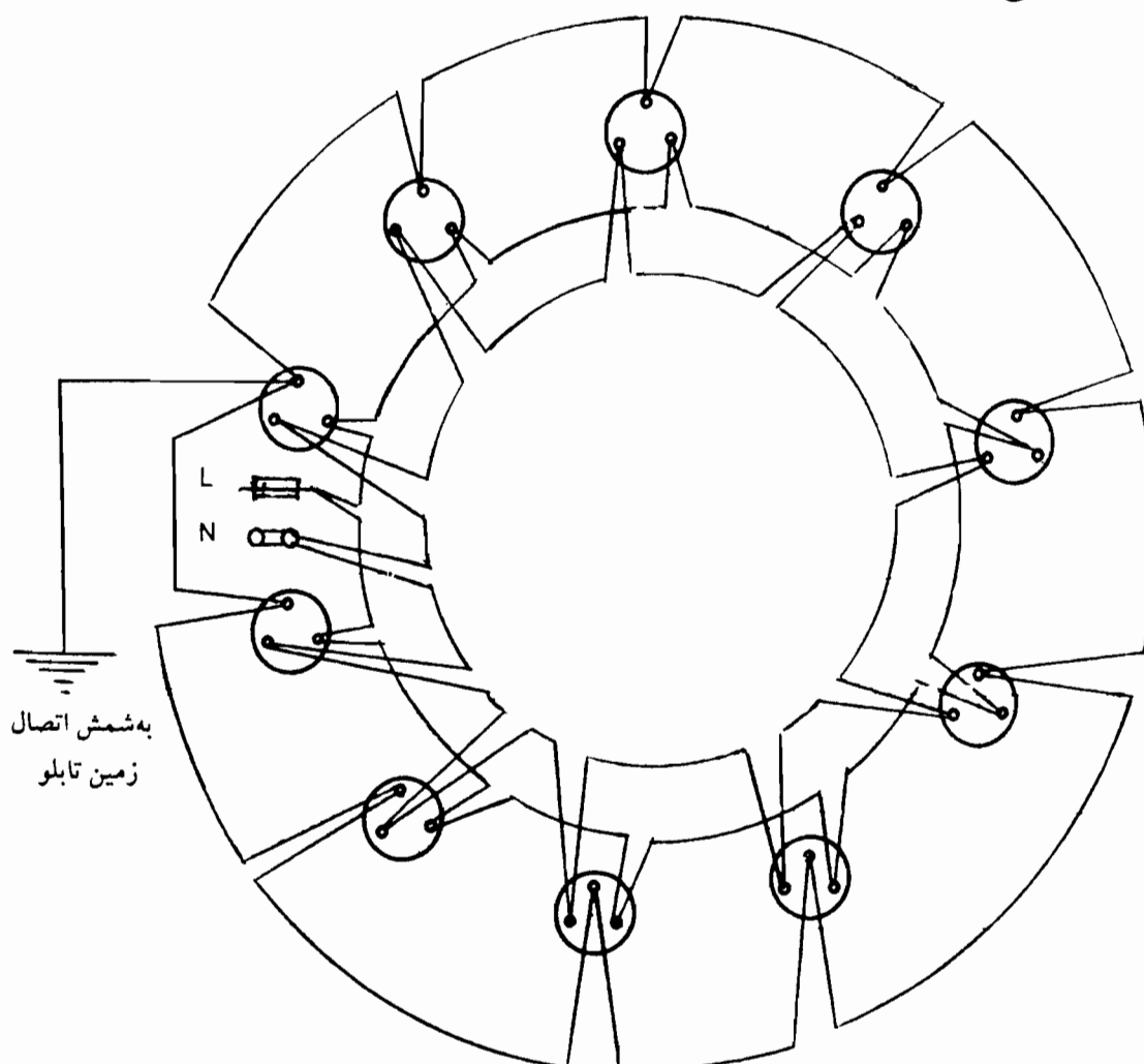
شکل ۲-۳ سیستم سیمکشی حلقوی مدار پریزها.
