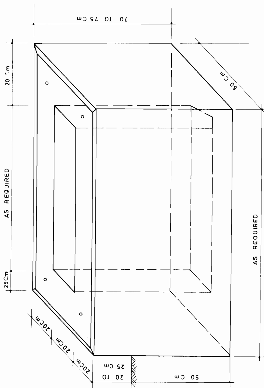
شکل ۲۰-۵. سکوی مخصوص نصب تابلوهای توزیع نیروی برق قابل نصب در فضای باز
