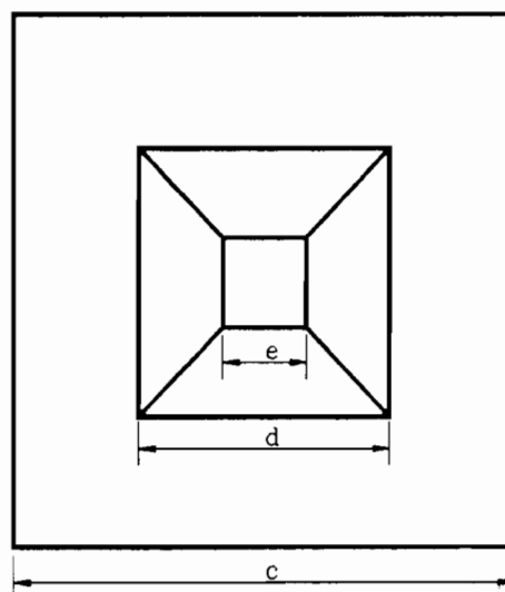
پلان نمونه فونداسیون بتنی پیش ساخته شکل ۶-۱۳
