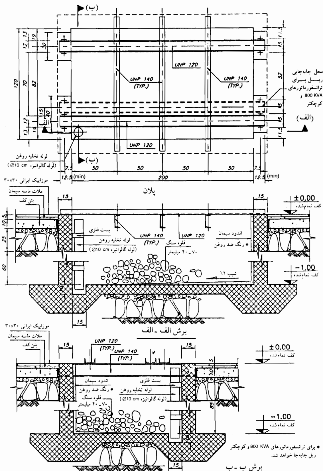
شکل ۱-۱ نمونه جزییات حوضچه روغن و ریل گذاری ترانسفورماتور برابر استاندارد وزارت نیرو - امور برق.
